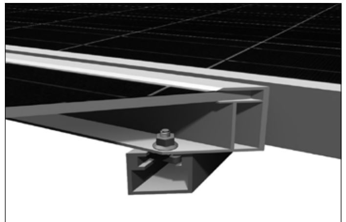
Beispiel 2 – Verschraubung direkt
