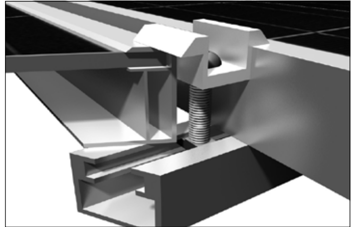
Beispiel 1 – Klemmflügel
